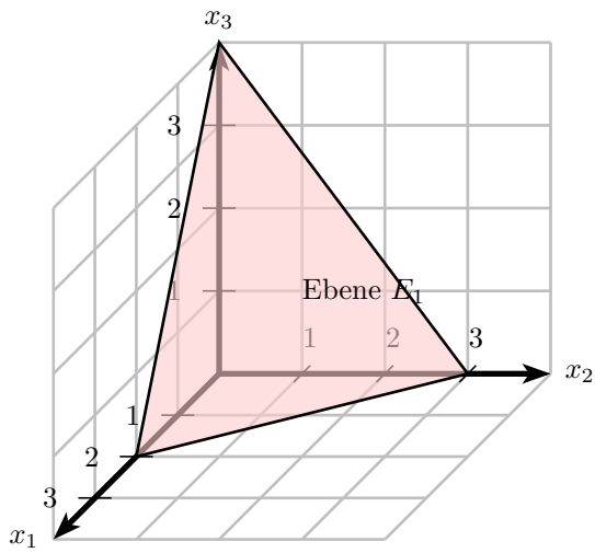
Abb. 1: E_1 : 6x_1 + 4x_2 + 3x_3 = 12
