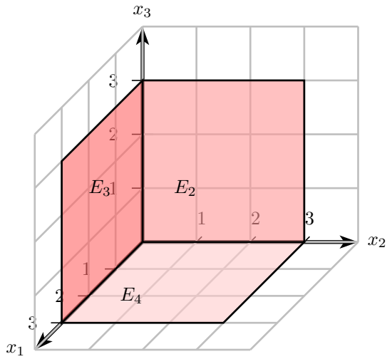
Abb. 2: E_2 : x_1 = 0 ; E_3 : x_2 = 0 ; E_4 : x_3 = 0
